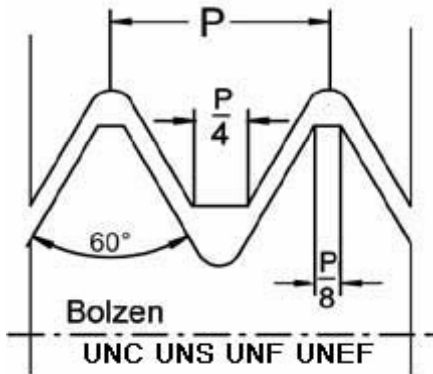
UNC, UNS, UNF, UNEF Gewinde
