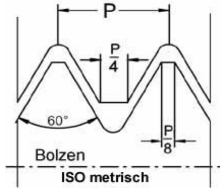
M und MF Gewinde
